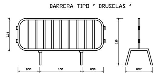
BARRERA TIPO "BRUSELAS"
