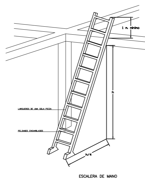
ESCALERA DE MANO
