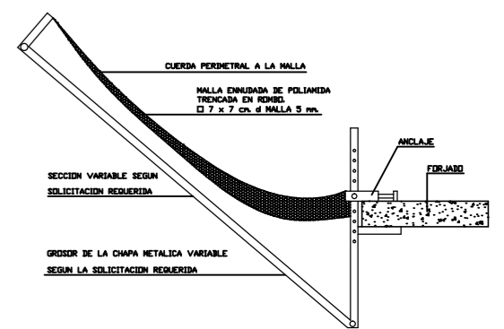
HORCON SIMPLE MARCA ALBO
