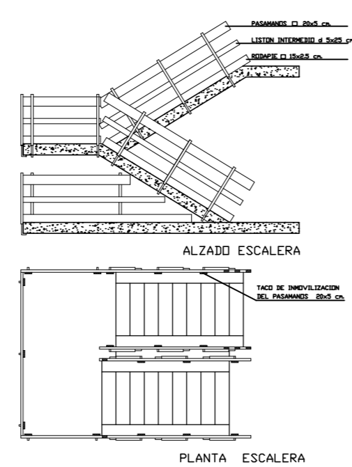
PLANTA ESCALERA
