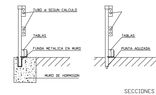
SECCIONES
