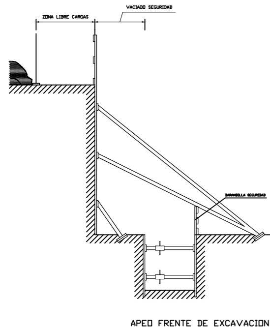
APEO FRENTE DE EXCAVACION
