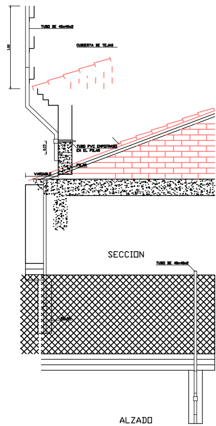
MAQUESINA DE SEGURIDAD
